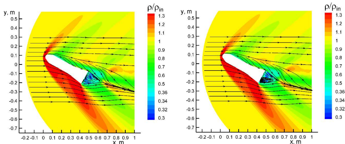
Рис. 6. Уровни плотности и линии тока для моментов времени, отличающихся на 0.014 с в сечении z = 0 , моделирование (вариант 2)
