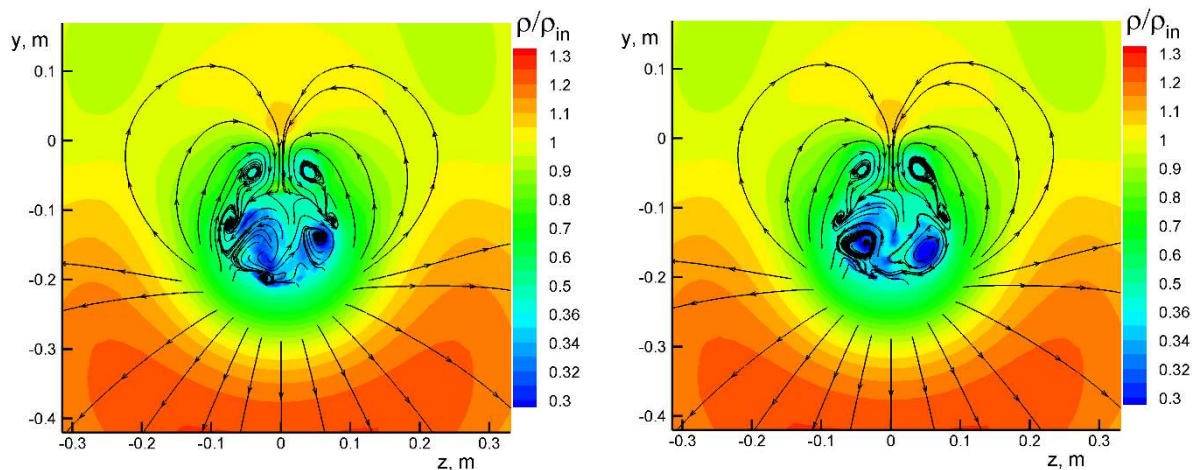
Рис. 8. Уровни плотности и линии тока для моментов времени, отличающихся на 0.014 с в сечении x = 0.491801 м, моделирование (вариант 2)
