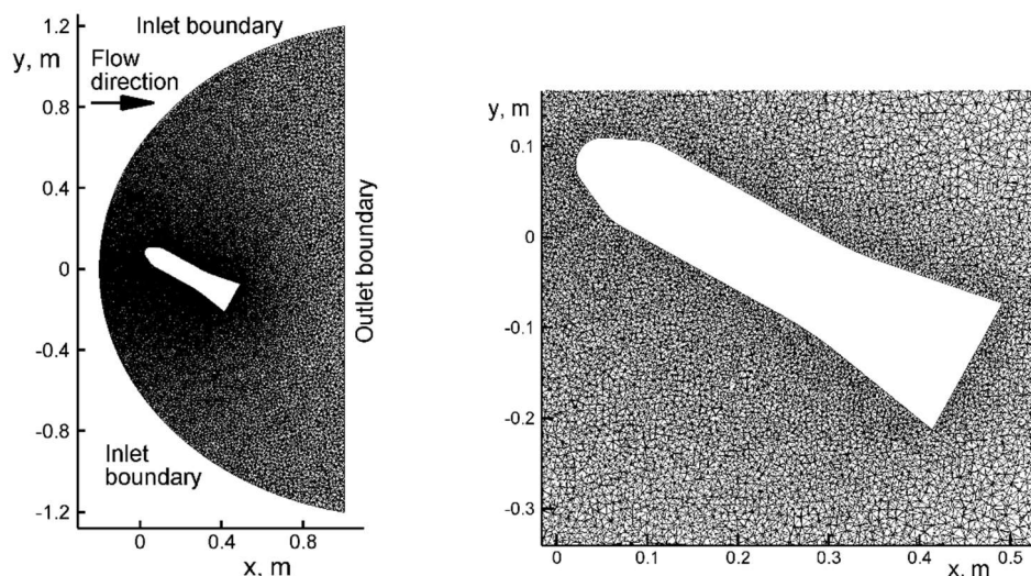
Рис. 2. Расчетная область и тетраэдральная сетка, построенная Gmsh в сечении z = 0 , слева общий вид, справа фрагмент
