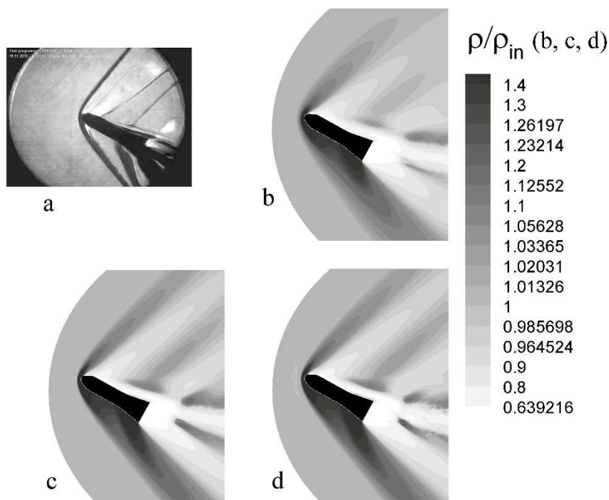
Рис. 4. Картины обтекания в сечении z = 0 : шлирен-изображение в эксперименте (а), уровни плотности при моделировании в вариантах 1–3 (b–d)
